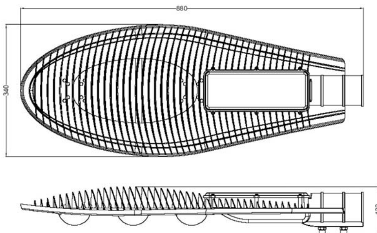
dimensions SCLA3-150 / 180
