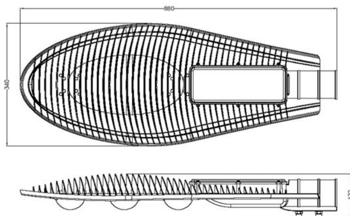
rozměry SCLA3-150 / 180
