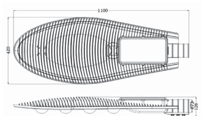
rozměry SCLA4-200 / 240
