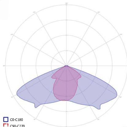
vyzařovací charakteristika
