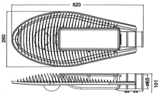
dimensions SCLA1-060 / 050 / 080
